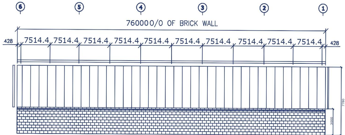
SIDE WALL FRAMING ELE.@ GL-A
