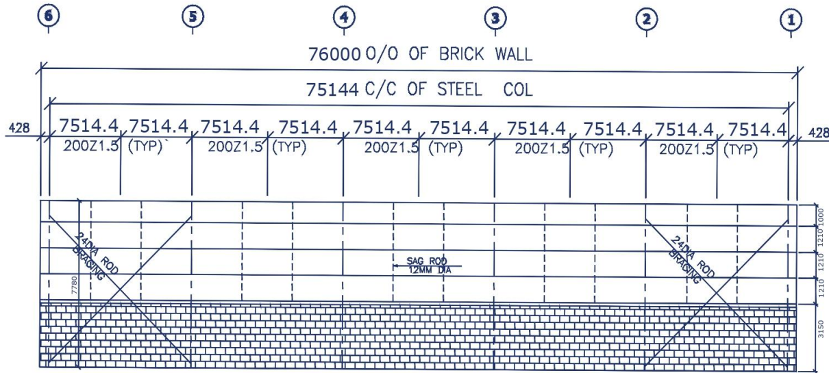
SIDE WALL FRAMING ELE.@ GL-A
